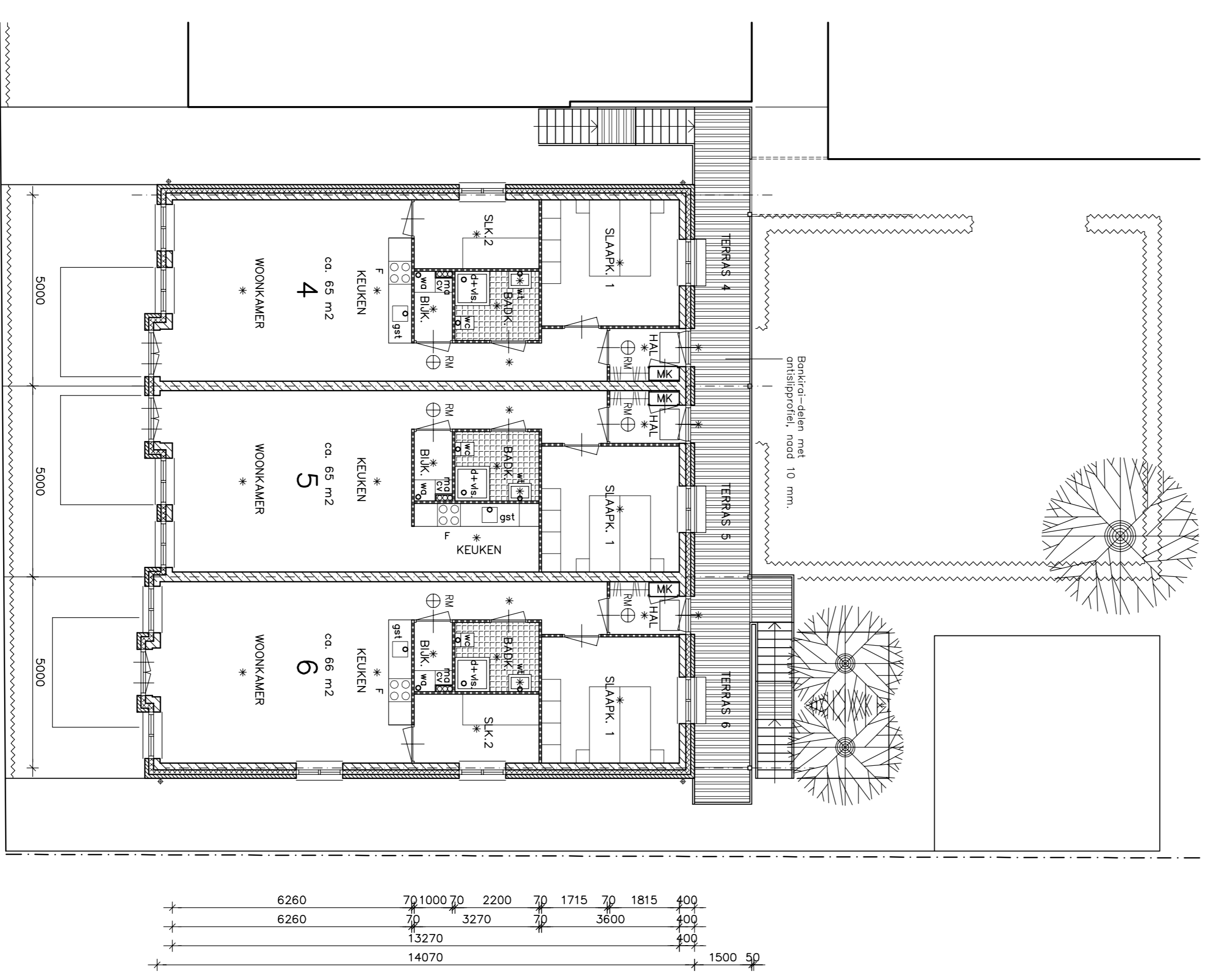
1e VERDIEPING
